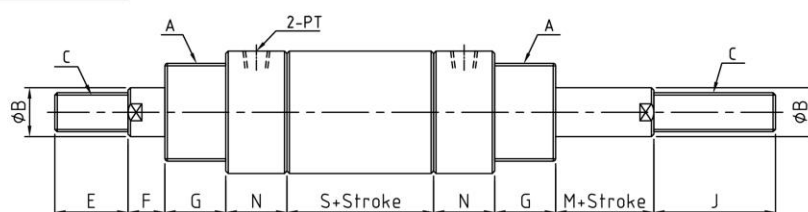
圓油雙軸型 RCD
