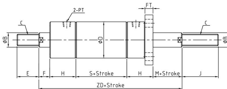
圓油FB雙軸型 RCD+FB
