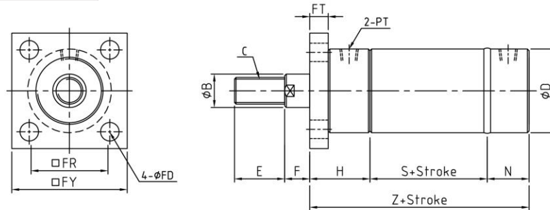
圓油FA雙軸型 RCD+FA
