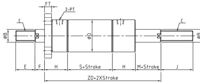
圓油FA雙軸型 RCD+FA
